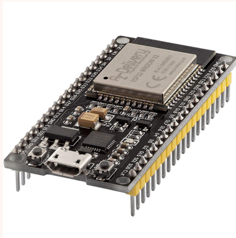
ESP 32 SDA: GPIO 21 | SCL: GPIO 22
